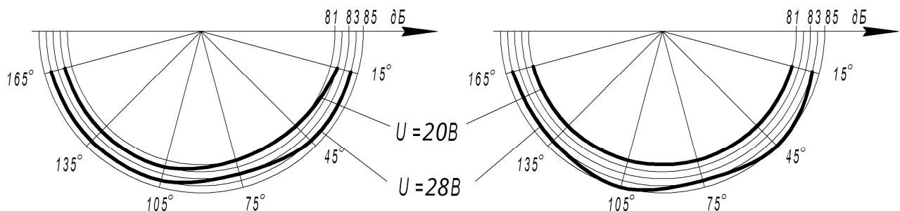
Рисунок 1 – Акустичні діаграми оповіщувача:
